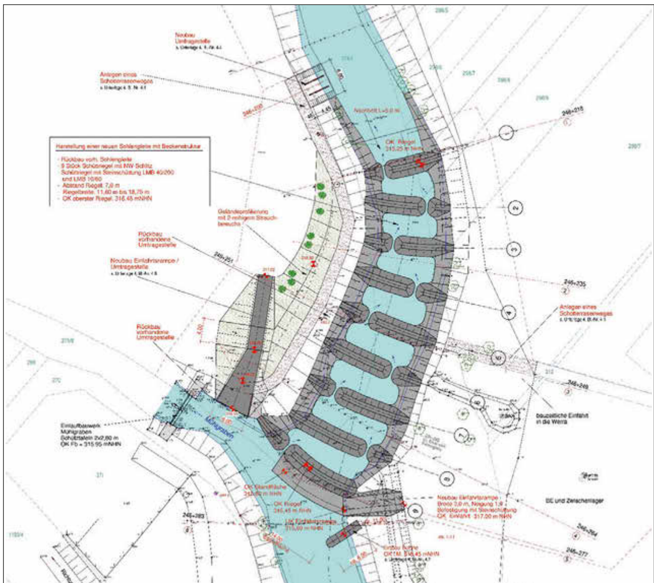
Abb. 1 Lageplan Sohlengleite, IB PROWA
