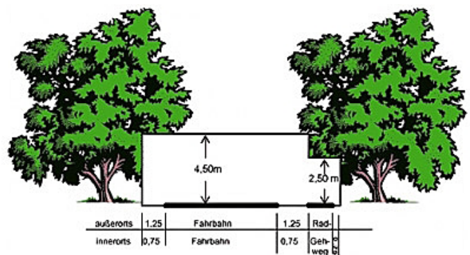
Lichtraumprofil
