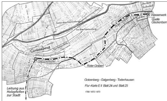
Die Flurkarte zur Wolfhager Wasserversorgung 1788 zeigt die Quelle des Glockenborns „An dem Todenhof“, wo der „Rote Graben“ beginnt, der am Sammelkeller endet. Von hier aus führten die Holzpfefen über das Flurstück „Zum Pfeiffen“ bis zum Hospital.
