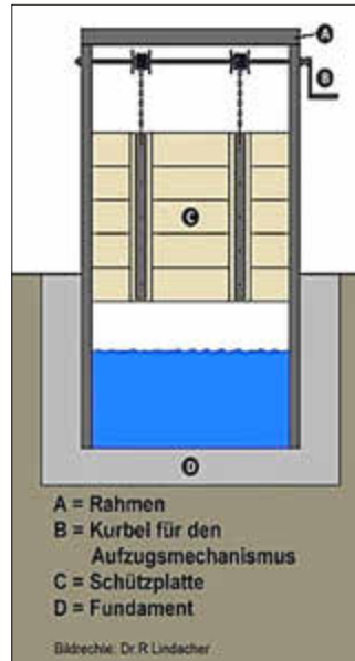
Abb. 1: Modell eines Kurbelschützes
