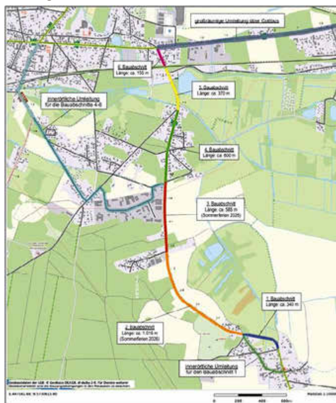
Bauabschnitte und innerörtliche Umleitung/Baumaßnahme L 50 zwischen Hänchen und Kolkwitz
