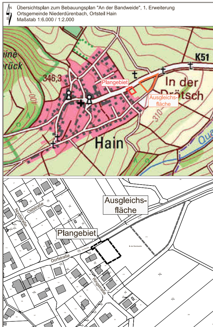
Übersichtsplan zum Bebauungsplan „An der Bandweide“, 1. Erweiterung Ortsgemeinde Niederdürenbach, Ortsteil Hain Maßstab 1:6.000 / 1:2.000
