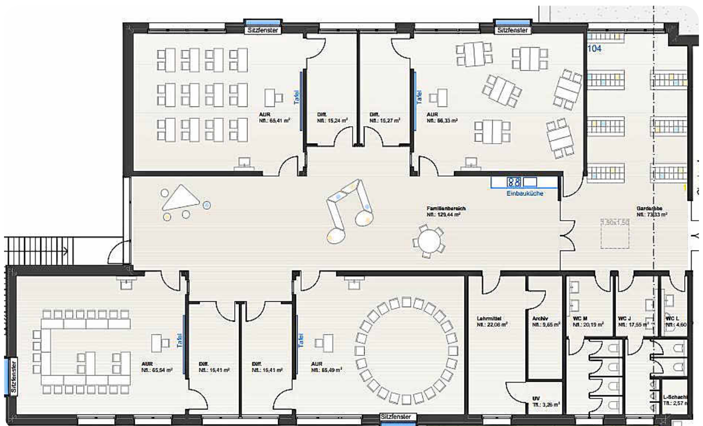
Grundriss von einem Schulbereich; 4 Klassenzimmer mit einer gemeinsamen Mitte
